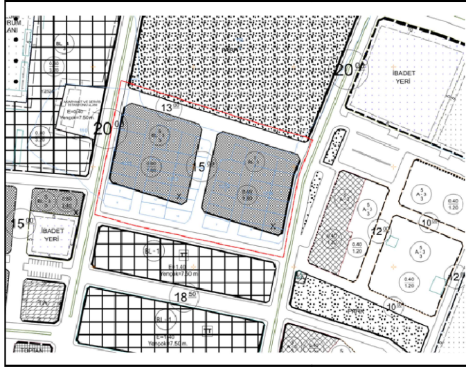
MEVCUT PLAN
