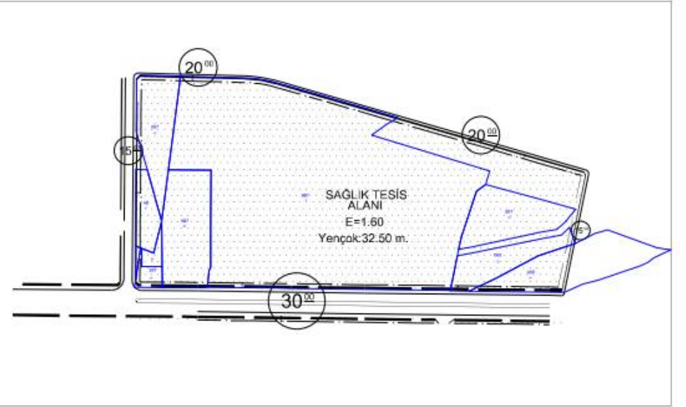
ÖNERİ PLAN
