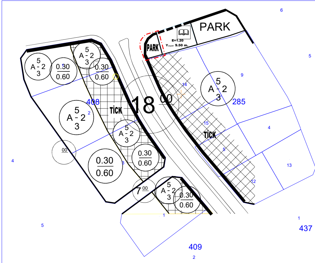
MEVCUT PLAN
